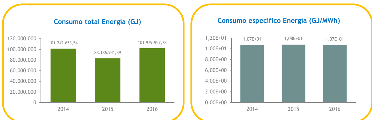
Gráfico 5. Evolución anual de consumo total y específico de energía en C.N.Cofrentes. Periodo 2014-2016.
