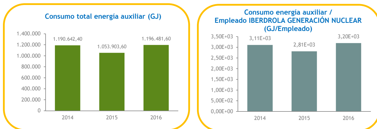
Gráfico 10. Evolución anual de consumo total y específico de energía auxiliar por empleado de IBERDROLA GENERACIÓN NUCLEAR en C.N. Cofrentes. Periodo 2014-2016.
