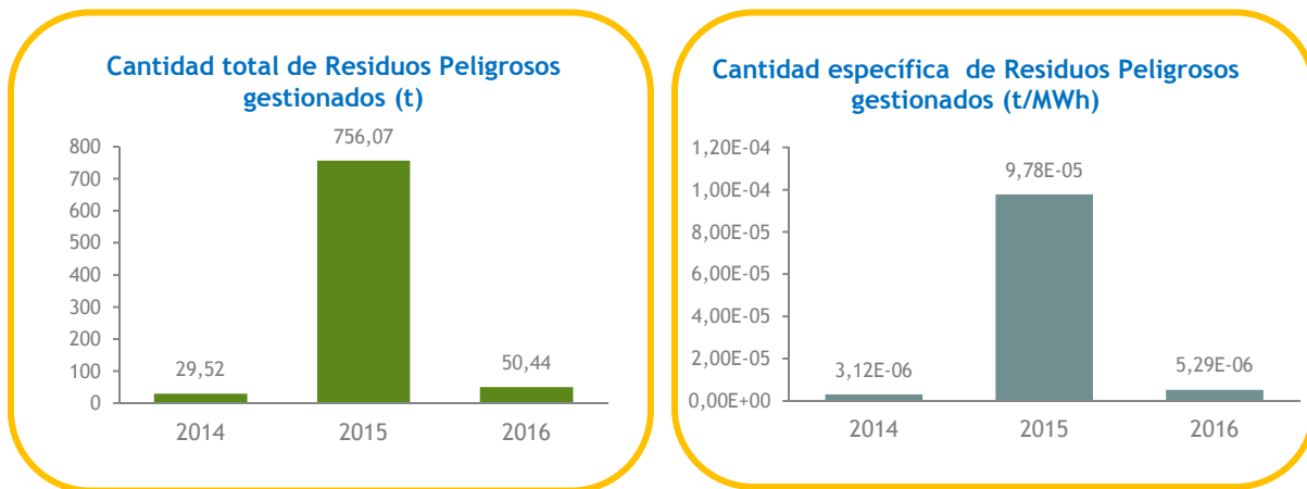
Gráfico 32. Evolución anual de la gestión total y específica de residuos peligrosos. Período 2014-2016.
