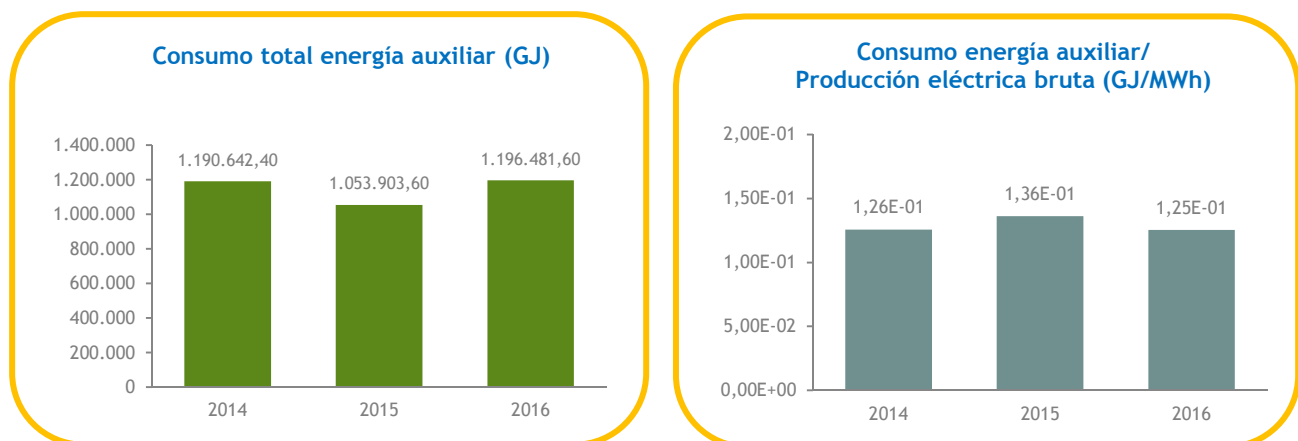
Gráfico 9. Evolución anual de consumo total y específico de energía auxiliar en C.N. Cofrentes. Periodo 2014-2016.
