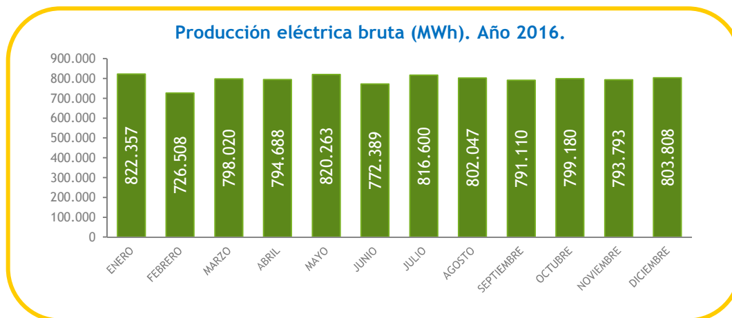
Gráfico 3. Evolución mensual de producción eléctrica bruta C.N. Cofrentes. Año 2016.
