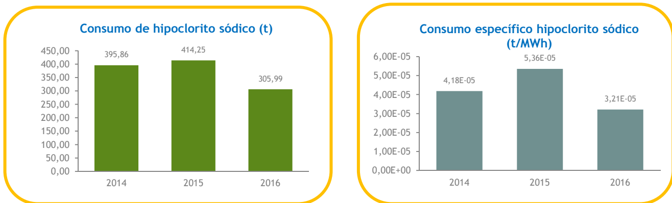
Gráfico 17. Evolución anual del consumo total y específico de hipoclorito sódico. Periodo 2014-2016.
