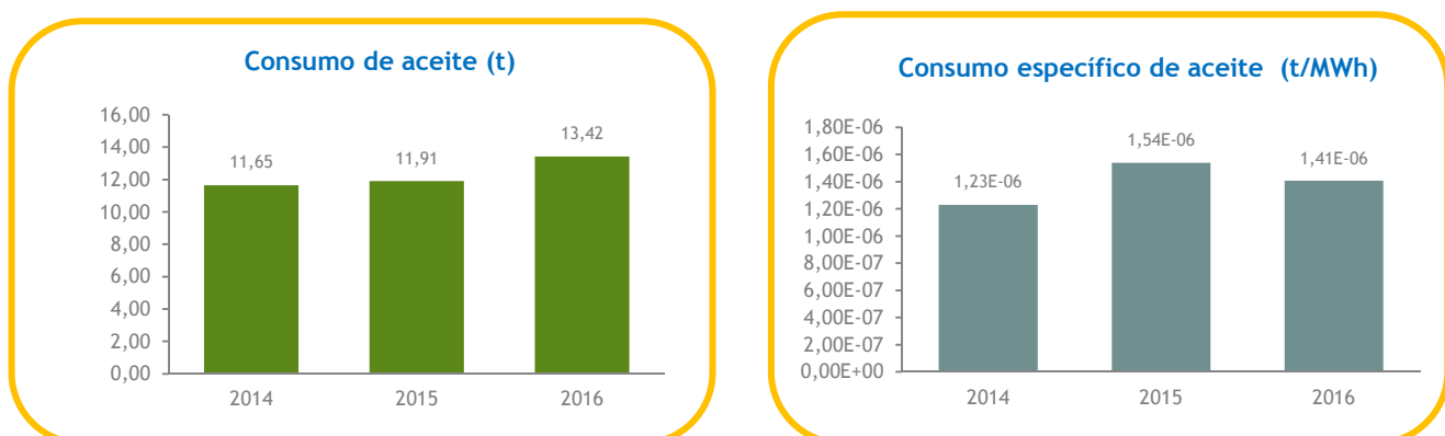
Gráfico 19. Evolución anual del consumo total y específico de aceite. Periodo 2014-2016.
