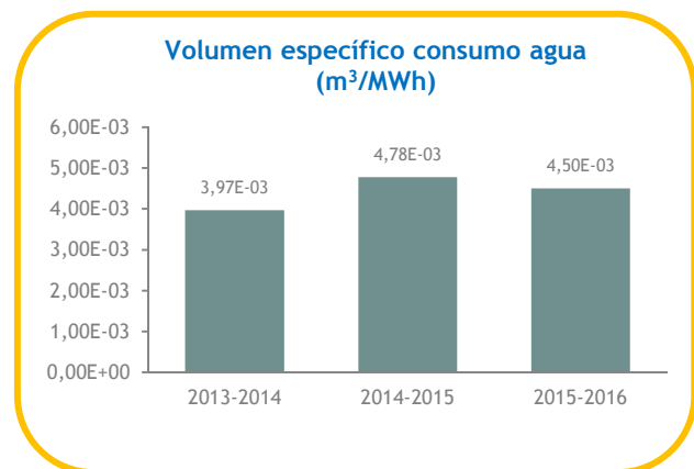
Gráfico 13. Evolución anual del Volumen total y específico de consumo de agua procedente de la Fuente Grande. Periodo años hidrológicos 2013-2014, 2014-2015 y 2015-2016
