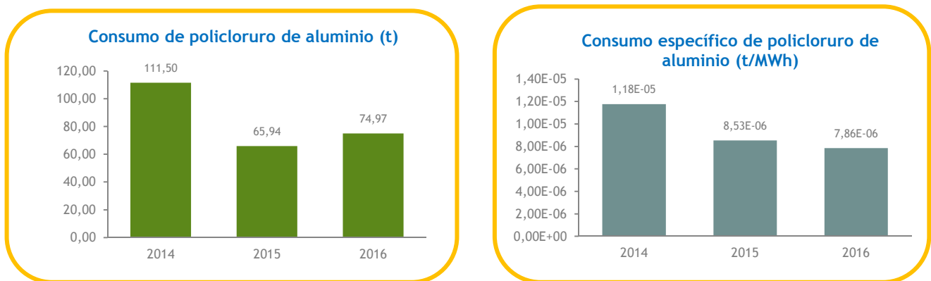
Gráfico 18. Evolución anual del consumo total y específico de policloruro de aluminio. Periodo 2014-2016.
