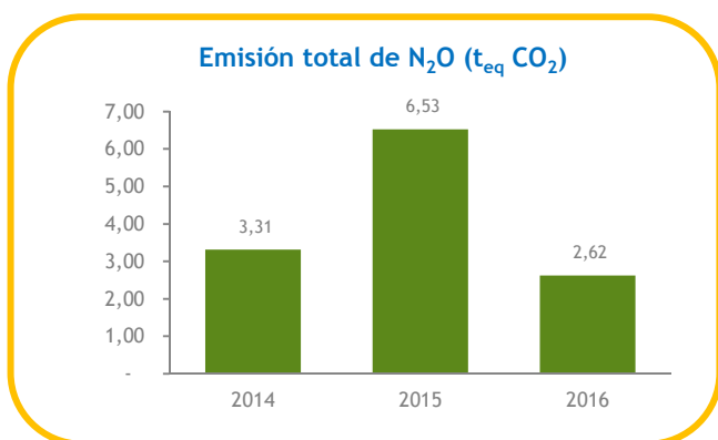
Gráfico 28. Evolución anual de la emisión total y específica de N 2 O. Periodo 2014-2016.
