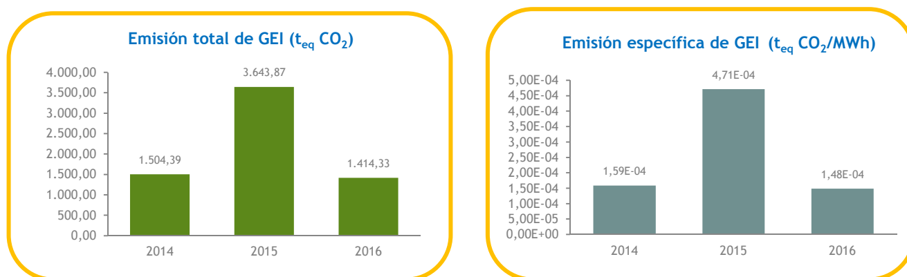
Gráfico 25. Evolución anual de la emisión total y específica de gases de efecto invernadero GEI. Periodo 2014-2016.
