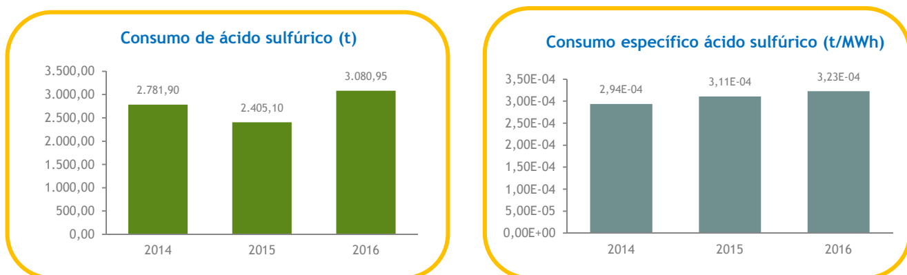
Gráfico 15. Evolución anual del consumo total y específico de ácido sulfúrico. Periodo 2014-2016.
