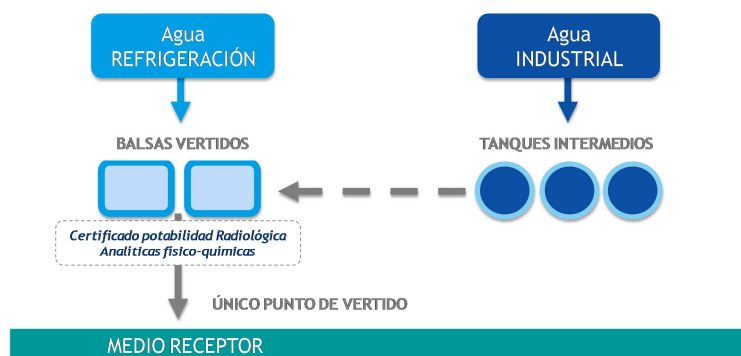
Figura 8. Esquema Sistema de Vertidos C.N. Cofrentes.
