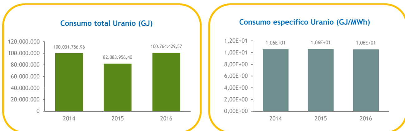
Gráfico 6. Evolución anual de consumo total y específico de Uranio en C.N.Cofrentes. Periodo 2014-2016.
