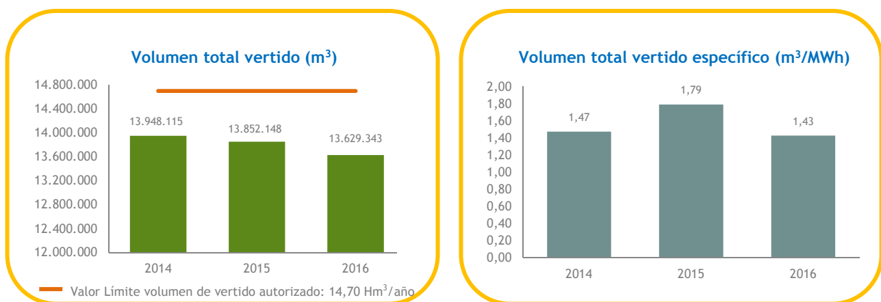
Gráfico 20. Evolución anual del volumen total y específico de vertido en C.N. Cofrentes. Periodo 2014-2016.
