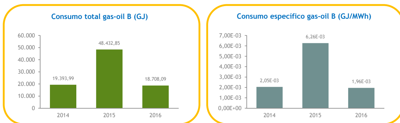
Gráfico 7. Evolución anual de consumo total y específico de gas-oil B en C.N. Cofrentes. Periodo 2014-2016.
