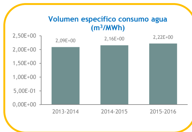
Gráfico 12. Evolución anual del volumen total y específico de consumo de agua procedente del Embalse de Embarcaderos. Periodo años hidrológicos 2013-2014, 2014-2015 y 2015-2016.
