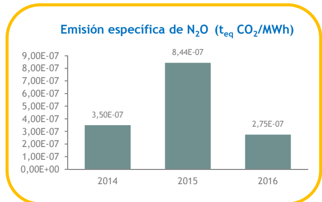
Gráfico 28. Evolución anual de la emisión total y específica de N 2 O. Periodo 2014-2016.
