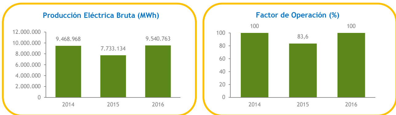
Gráfico 4. Evolución producción eléctrica bruta y factor de operación de C.N. Cofrentes. Periodo 2014-2016.
