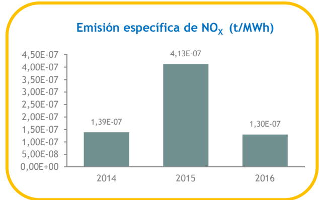
Gráfico 23. Evolución anual de la emisión total y específica de NO x . Periodo 2014-2016.
