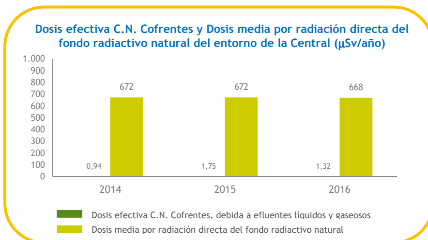
Gráfico 31. Comparativa de la dosis media anual por radiación directa del fondo radiactivo natural y dosis efectiva acumulada al público de C.N. Cofrentes. Periodo 2014-2016.
