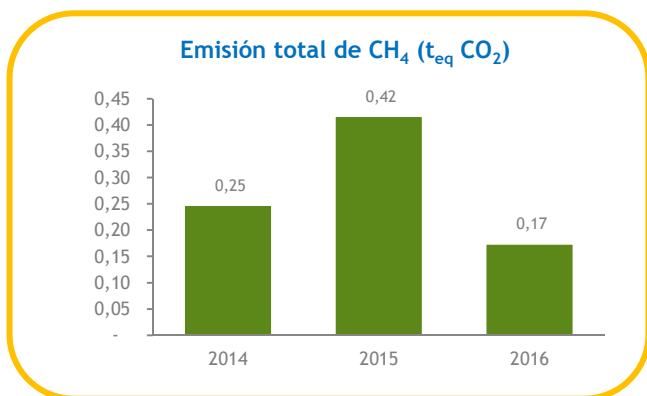
Gráfico 27. Evolución anual de la emisión total y específica de CH 4 . Periodo 2014-2016.
