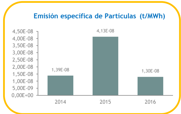
Gráfico 24. Evolución anual de la emisión total y específica de Partículas. Periodo 2014-2016.
