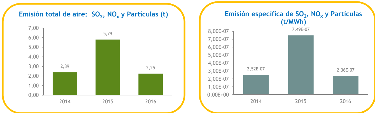
Gráfico 21. Evolución anual de la emisión total y específica al aire. Periodo 2014-2016.
