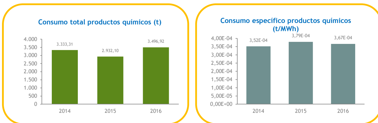
Gráfico 14. Evolución anual de consumo total y específico de productos químicos en C.N. Cofrentes. Periodo 2014-2016.
