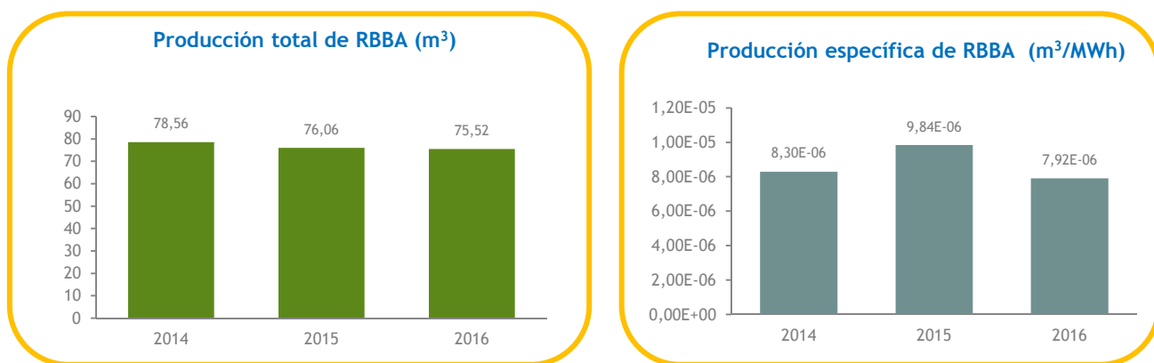
Gráfico 37. Evolución anual producción total y específica de RBBA en C.N. Cofrentes. Periodo 2014-2016.
