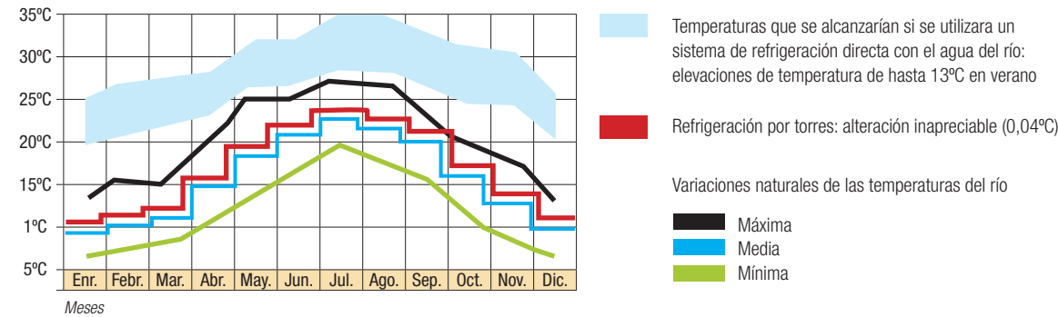
Comparación de incrementos de temperatura producidos en el río con y sin instalación de torres de refrigeración
