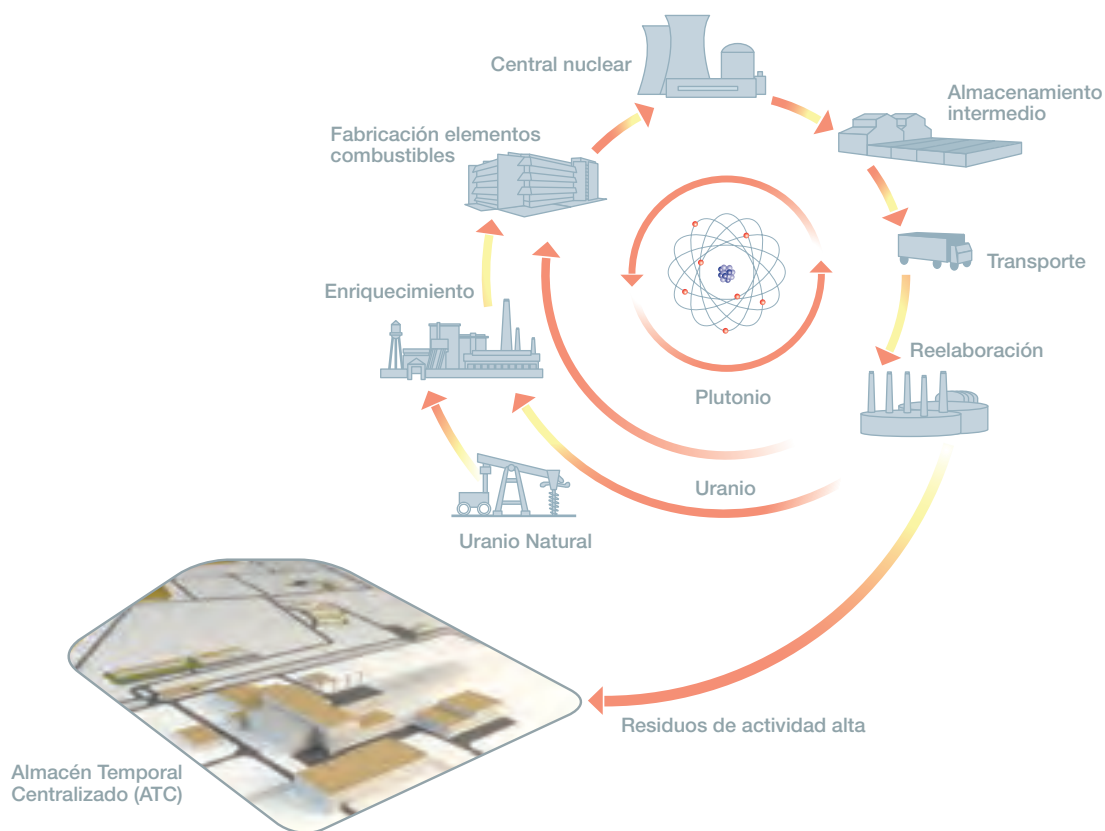
Esquema del ciclo cerrado del combustible
