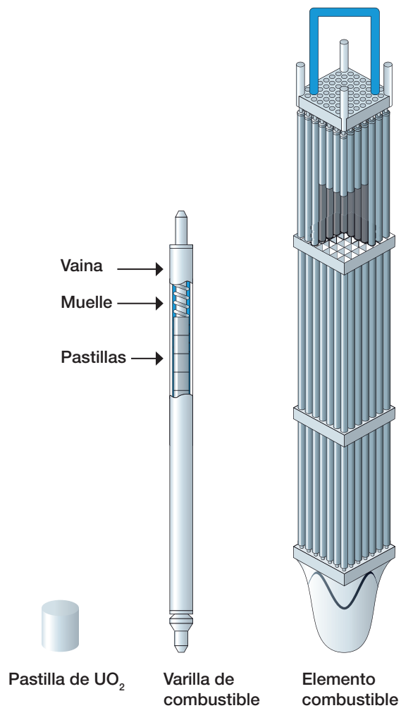
Composición de un elemento combustible
