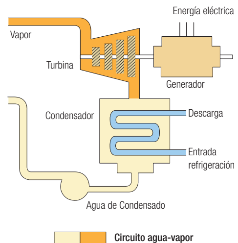
Esquema simplificado de la refrigeración de una central eléctrica convencional o nuclear
