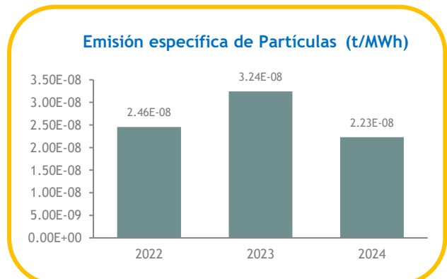
Gráfico 22. Evolución anual de la emisión total y específica de Partículas. Periodo 2022-2024.
