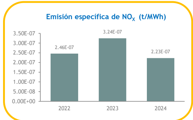
Gráfico 21. Evolución anual de la emisión total y específica de NO x . Periodo 2022-2024.
