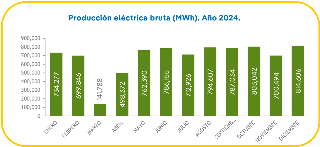
Gráfico 3. Evolución mensual de producción eléctrica bruta C.N. Cofrentes. Año 2024.
